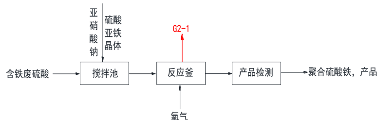
图 1.5.2-1 废硫酸处置生产聚合硫酸铁溶液工艺流程及产污环节
